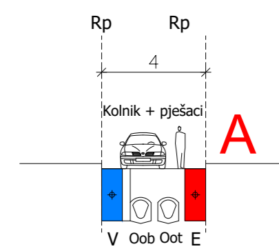
POPREČNI PROFIL PLANIRANE ULICE 'A' - m.1:200
